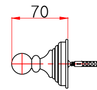
측면도
