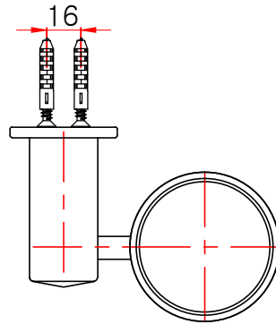
평(윗)면도
