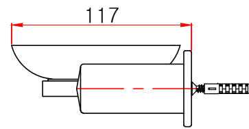
측면도
