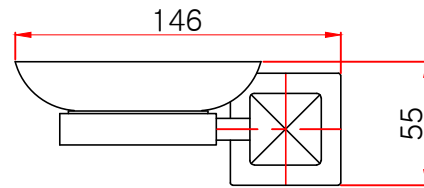
좌면도
