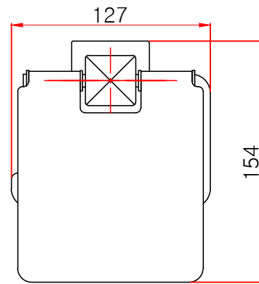
정면도
