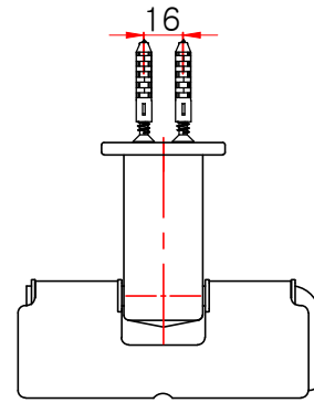
평(윗)면도
