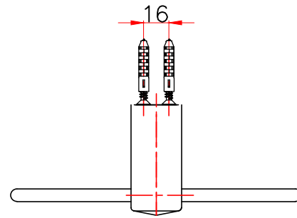
평(윗)면도
