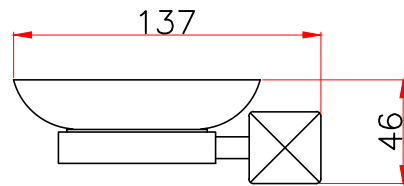
정면도
