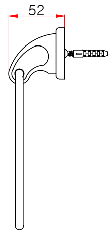
측면도
