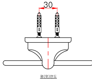
평(위)면도
