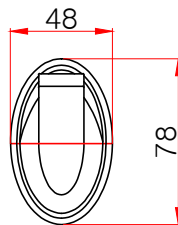
좌면도
