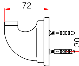
측면도
