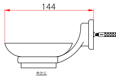
측면도
