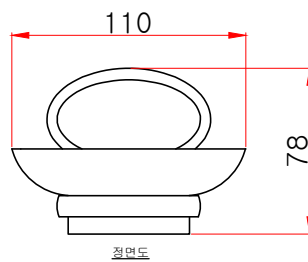
전면도
