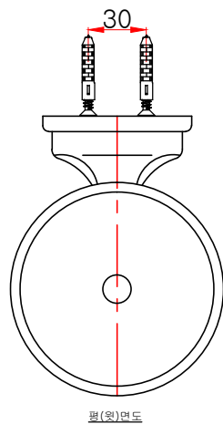
평(상)면도
