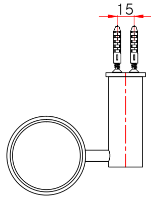
평(윗)면도
