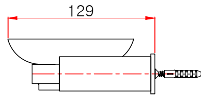
측면도
