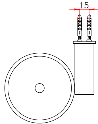
평(윗)면도
