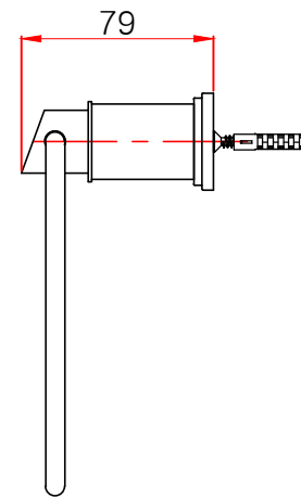
측면도
