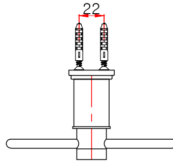
평(윗)면도
