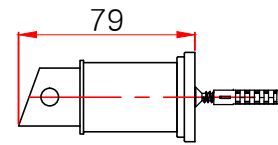
측면도
