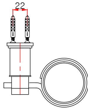
평(위)면도
