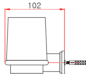
측면도
