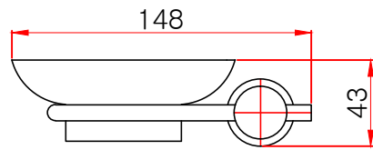
좌면도
