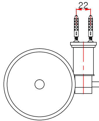
평(위)면도
