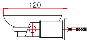
측면도
