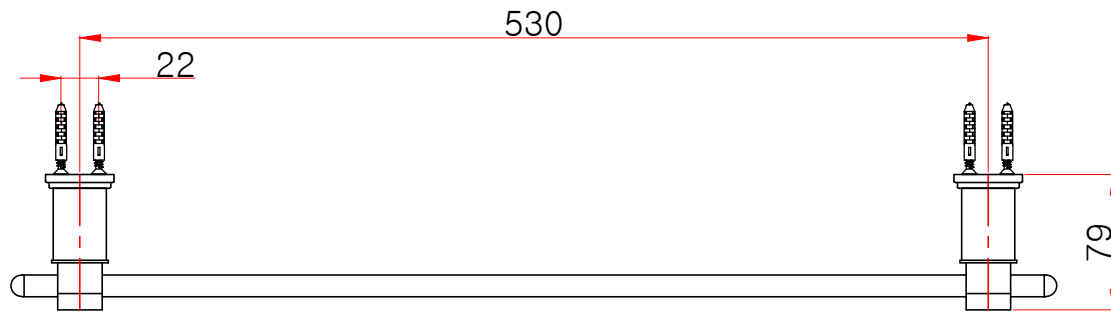
평(위)면도
