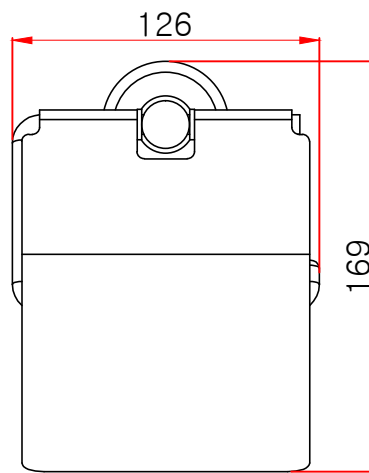
정면도
