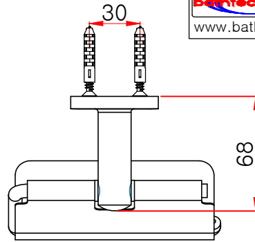
평(위)면도
