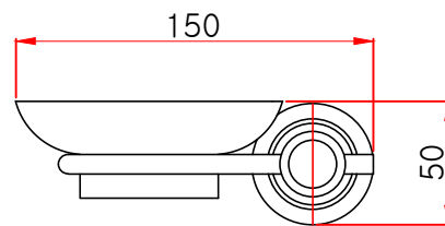
정면도
