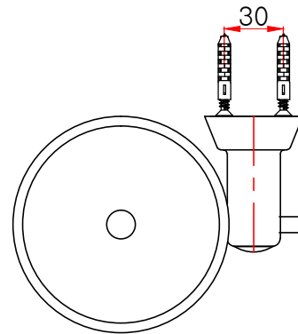
평(윗)면도
