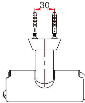
평(윗)면도
