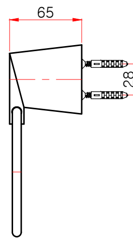
측면도
