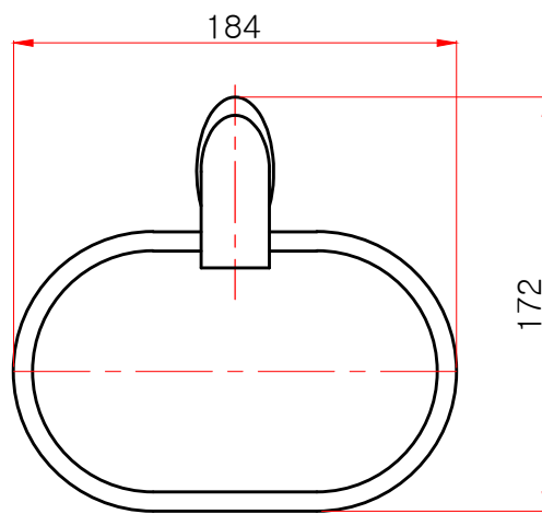
정면도
