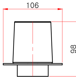
정면도
