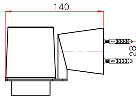
측면도
