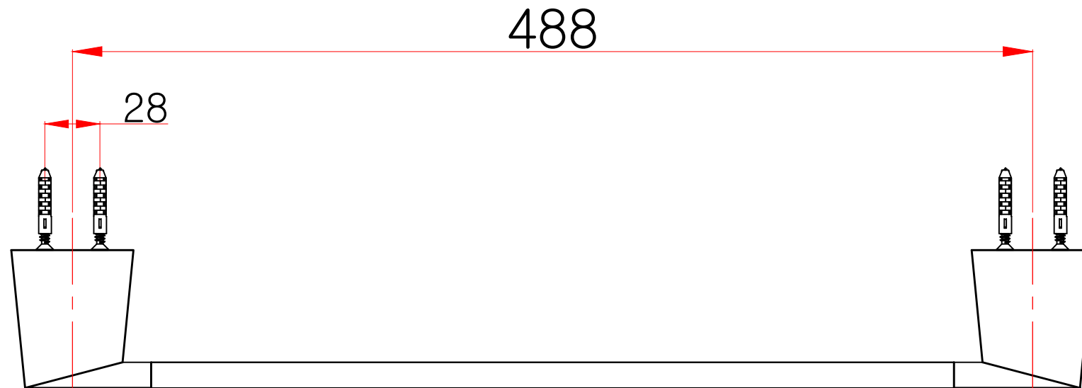
평(윗)면도
