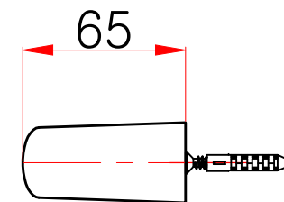
측면도
