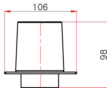
정면도
