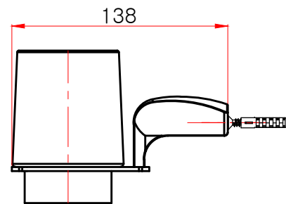
측면도
