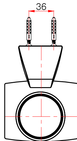
평(윗)면도
