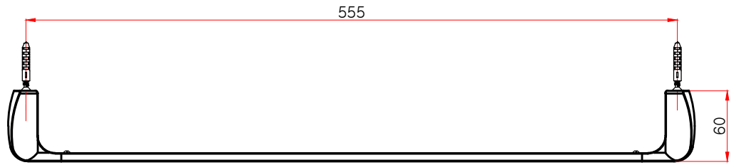
평(윗)면도
