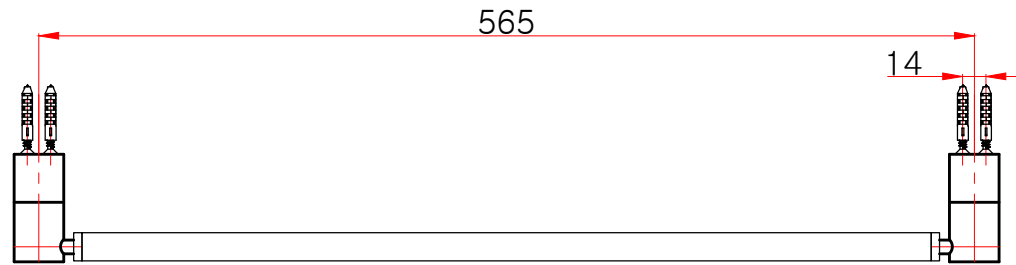
평(윗)면도
