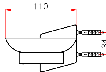
측면도
