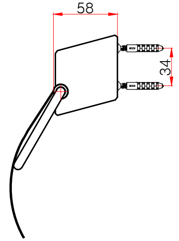
측면도
