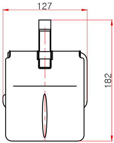
정면도
