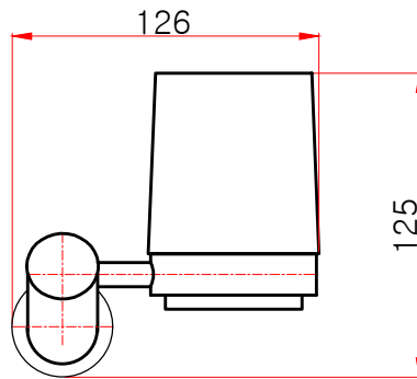
정면도
