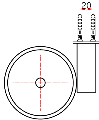
평(頂)면도
