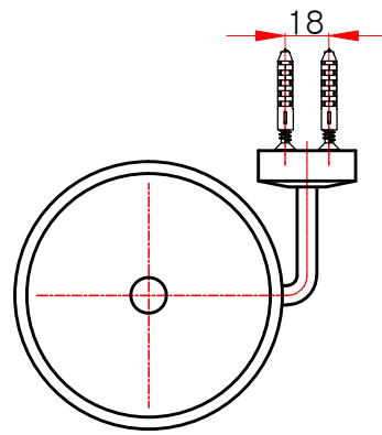
평(위)면도
