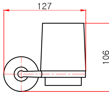
정면도
