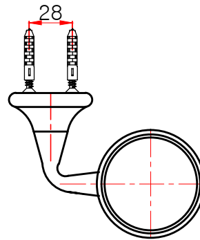
평(頂)면도
