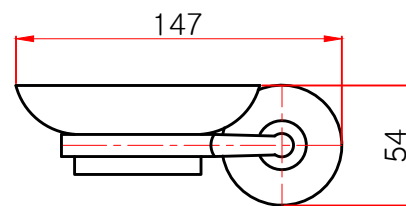
좌면도
