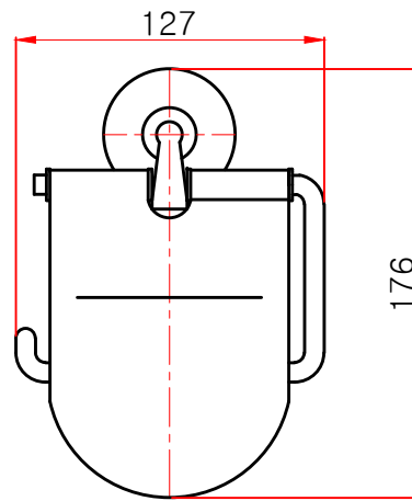
정면도
