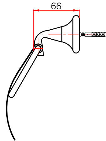
측면도
