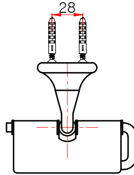
상면도
